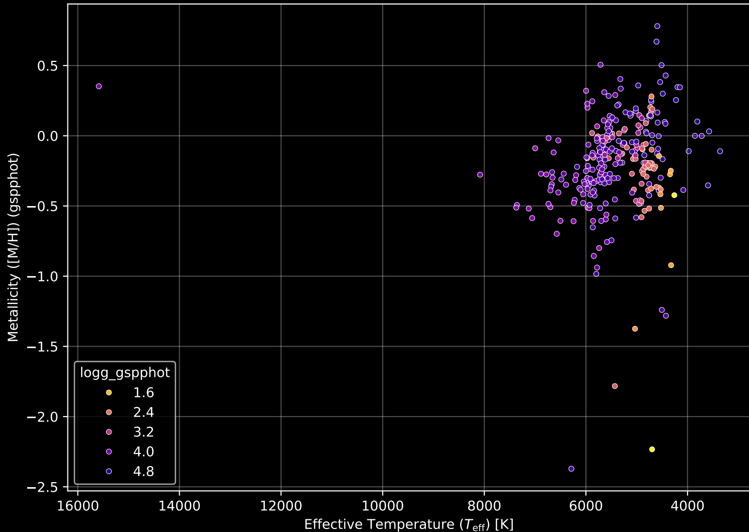
APOGEE DR17 Field: [057+35_MGA] Stellar Population Parameters (n= 294)
